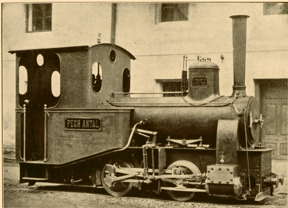
Gőzmozdony Hodrusbányán
