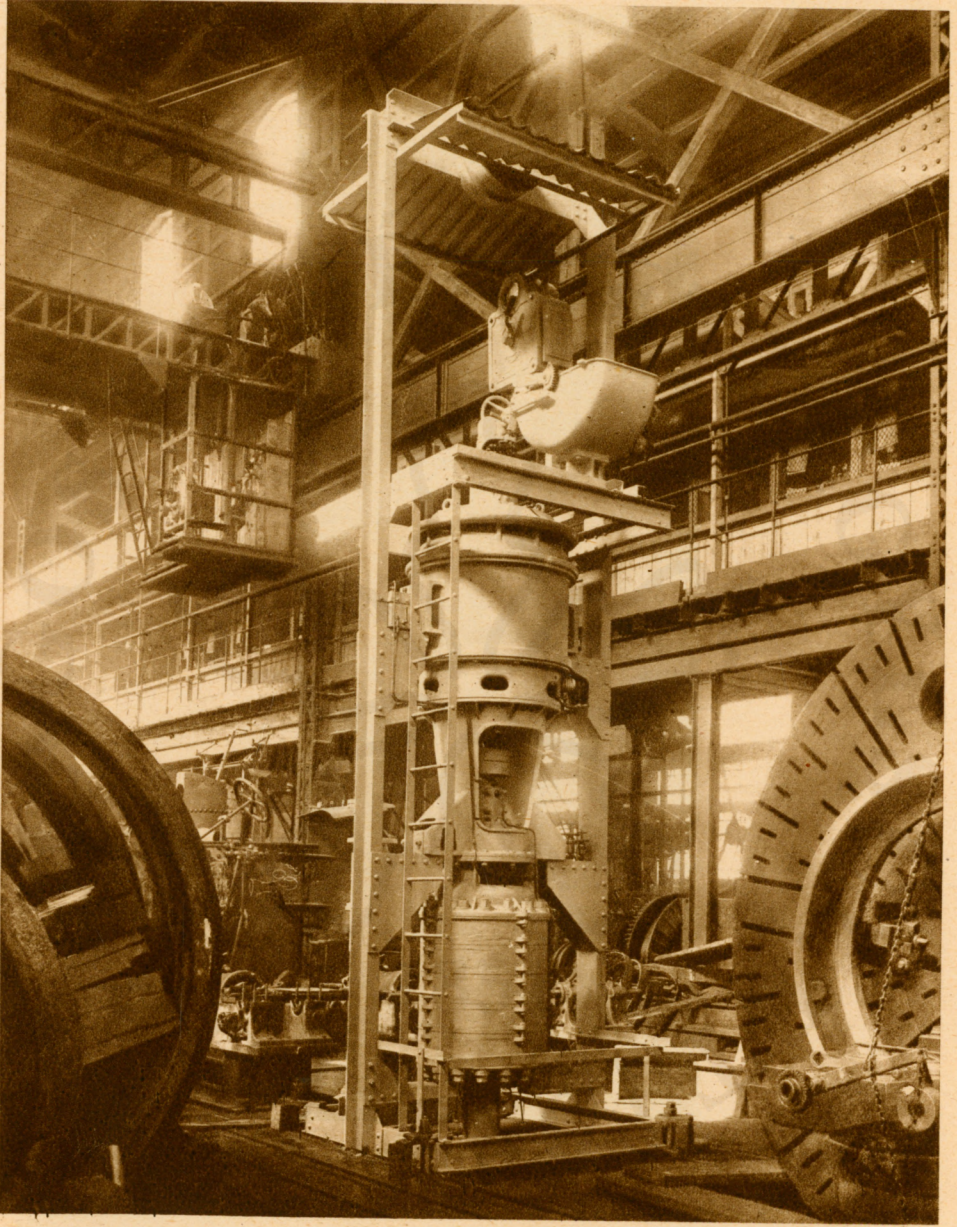
Függélyes aknaszivattyú.
