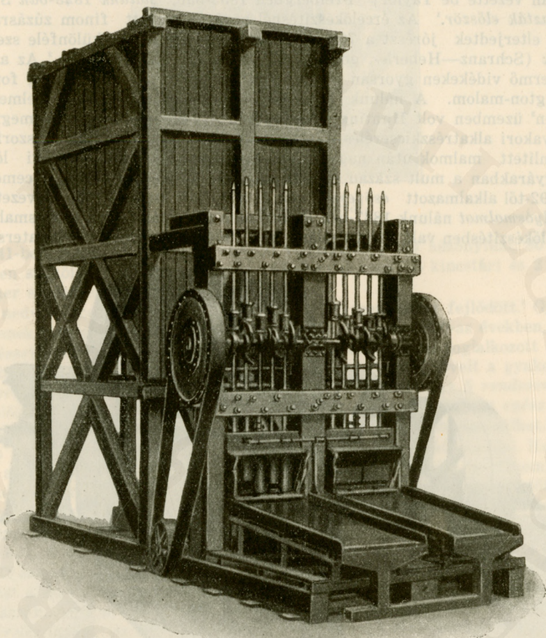
Tíznyilas kaliforniai zúzó
