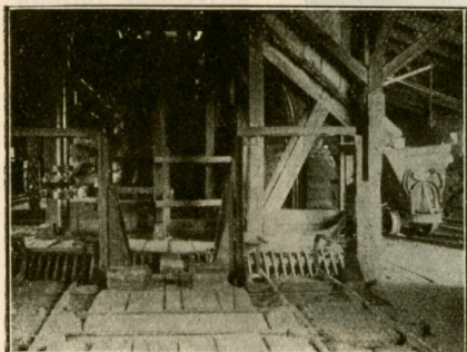
Ércbuktató lejtős rács.
