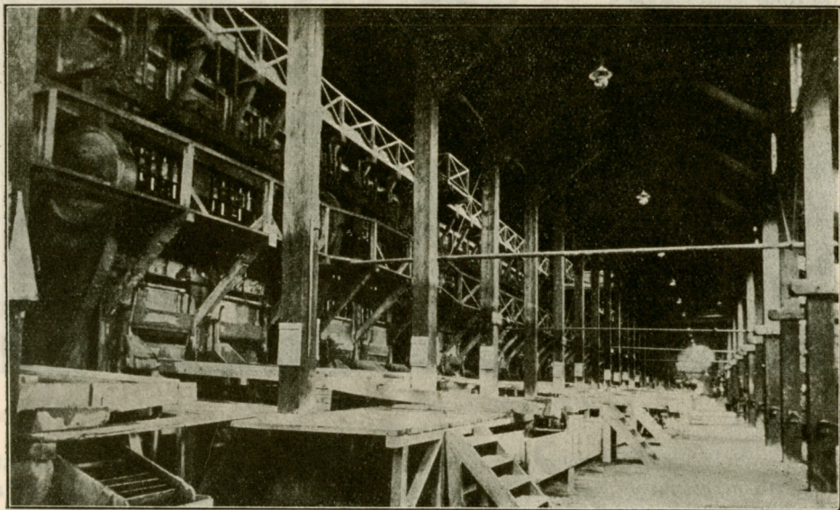
A rudai 12 apostol bányá központi ércelőkészítőműve Gurabárázán.
