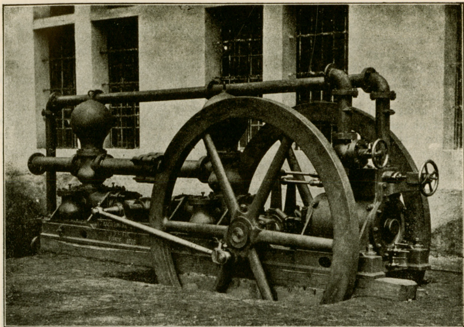
A selmeci Ferenc József-aknán 1878-ban felállított gőzszivattyú.
