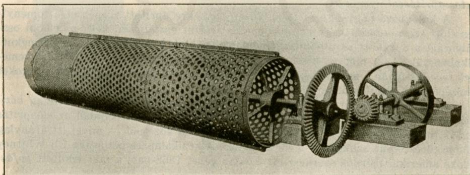
Osztályozódob.
