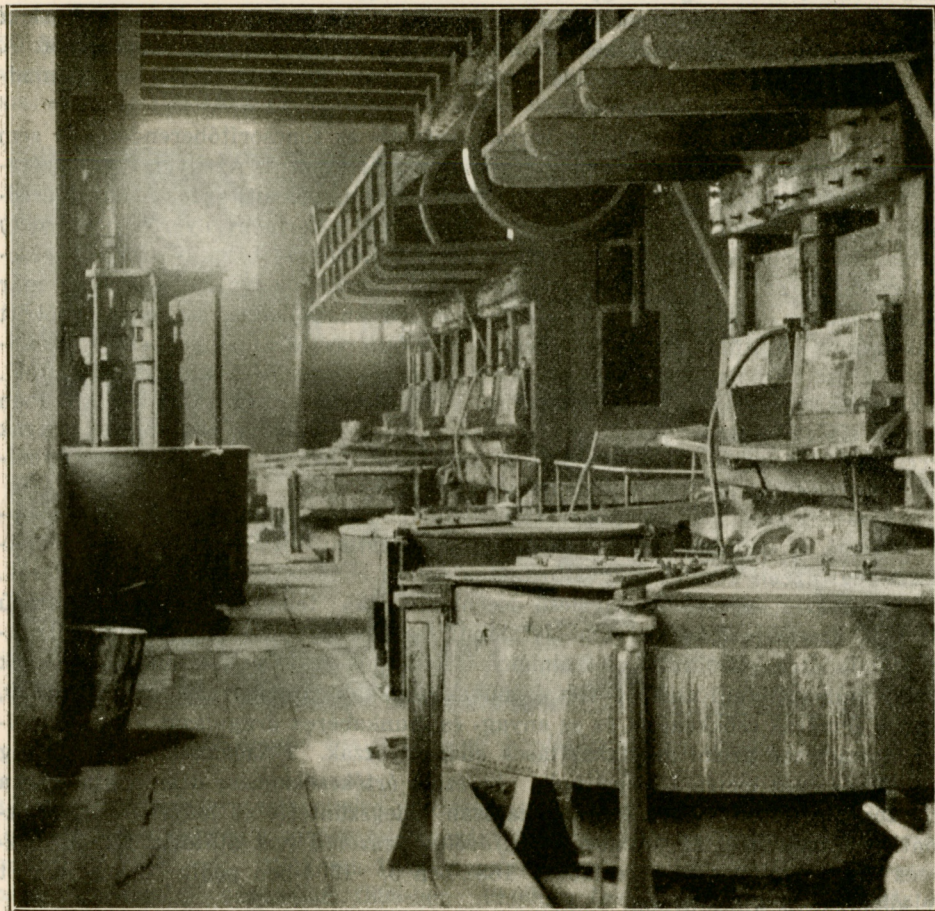
Boklevskij-féle amalgamátor Körmöcbányán.
