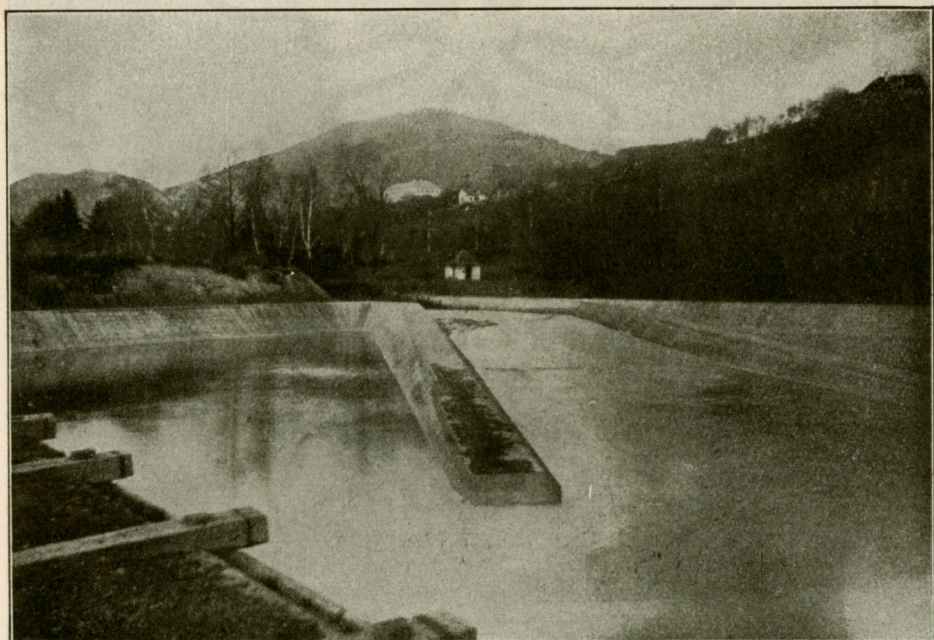
A körmöcbányai 1100 lóerős hidroelektromos erőközpont vízgyűjtőmedencéje.
