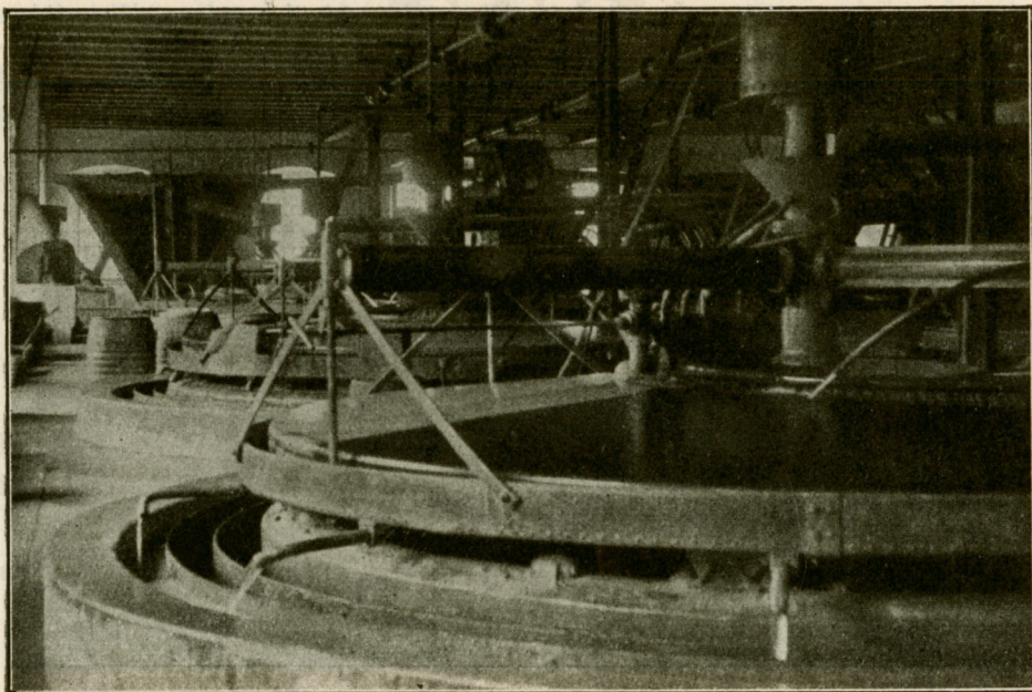
Bartsch-féle szér Körmöcbányán.
