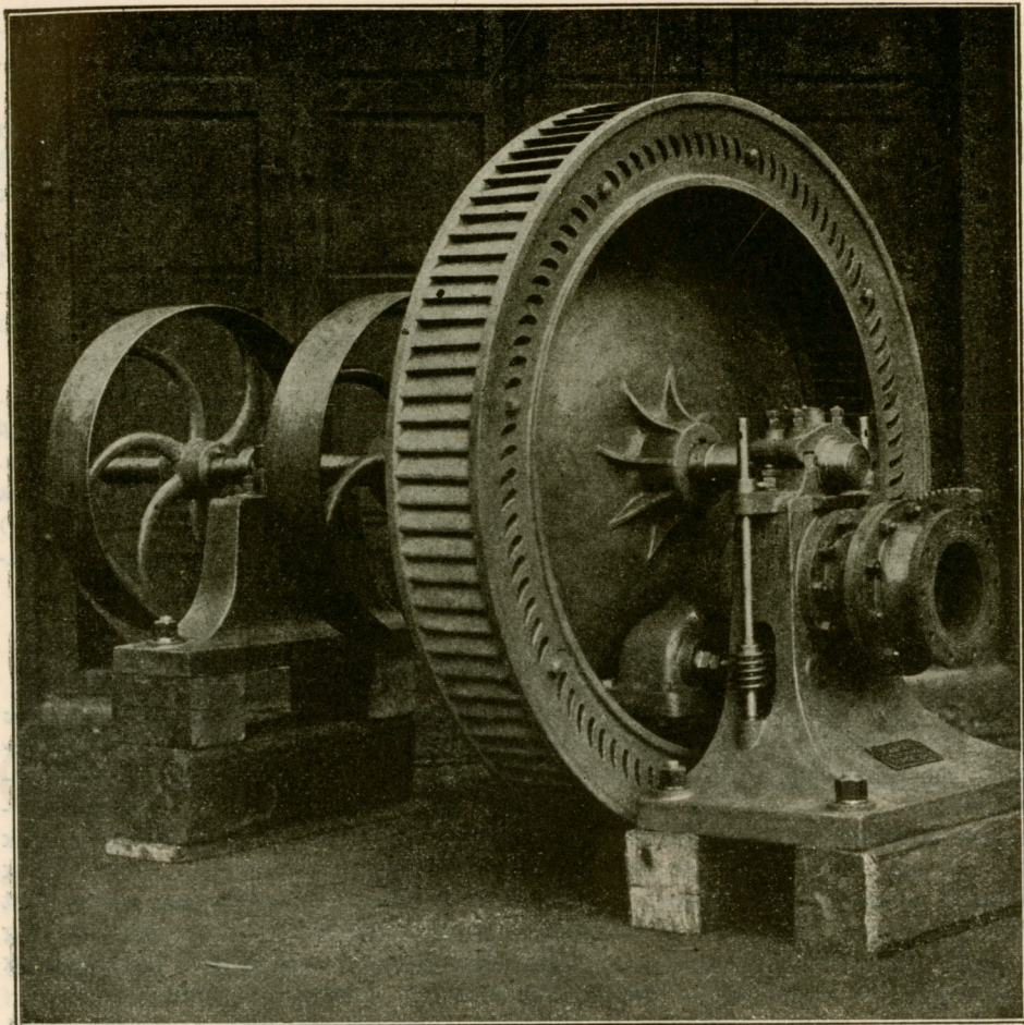
Girard-turbina Hodrusbányán.
