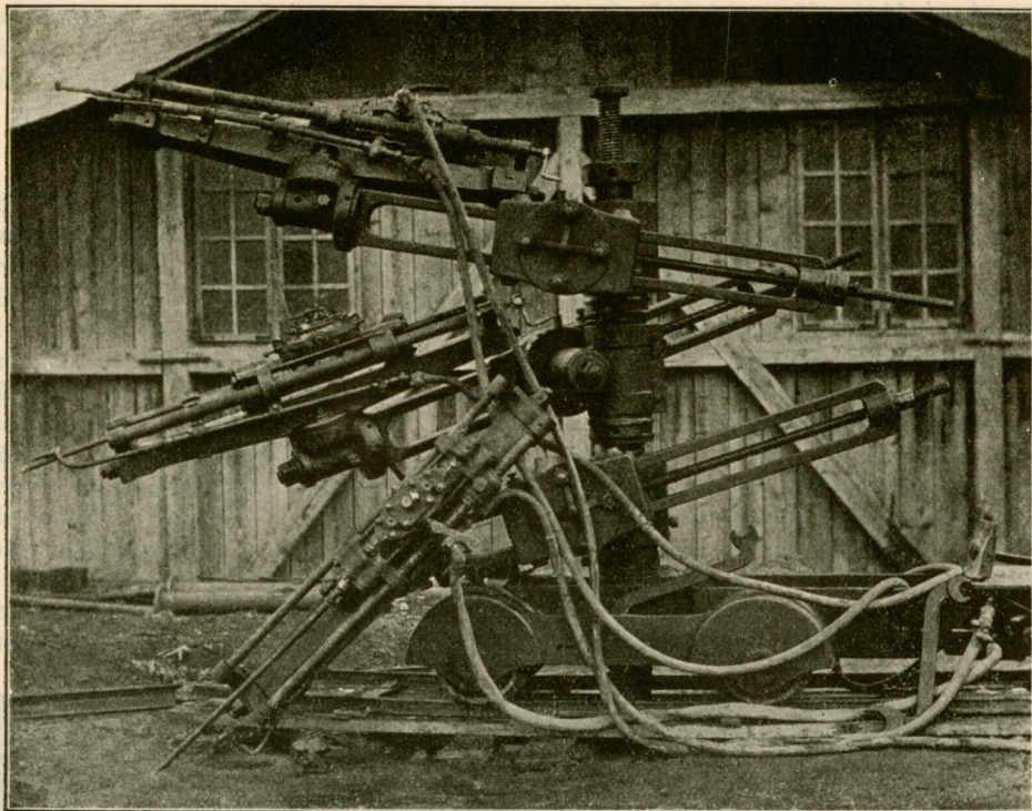
Broszmann—Kachelmann-féle kőzetfúrógépek Péch-féle állványon.
