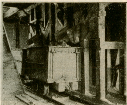
A pofástörőn feltört érc csüllékbe eresztése.
