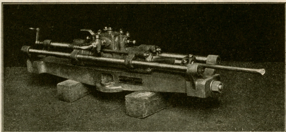
A selmeci II. József-altáró átlyukasztásánál 1874-ben használt Broszmann—Kachelmann-féle kőzetfúrógép.
