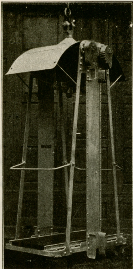
Régi (1880) és újabb típusú éreszállítókas.
