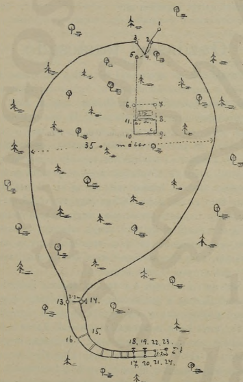
5. ábra. A maluzsinai szarvasbefogó vázlatos alaprajza. 1:50 mm. = 1 m.
