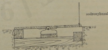
4. ábra. A vízszintes tengelyen mozgó hidlásszerű állás. 5 cm. = 1 m.
