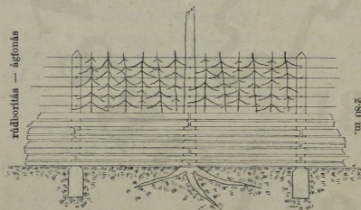
1. ábra. A kerítés. 1 cm. = 1 m.
