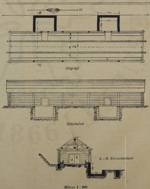
4. ábra. Istálló hosszanti fekvéssel bíró jászollal.
