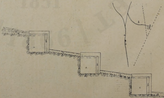
12. ábra. Fent: Földalatti csövek a tervrajza, mellyel a vizet a vályukhoz vezetik. Lent: A vályuk elhelyezése.
