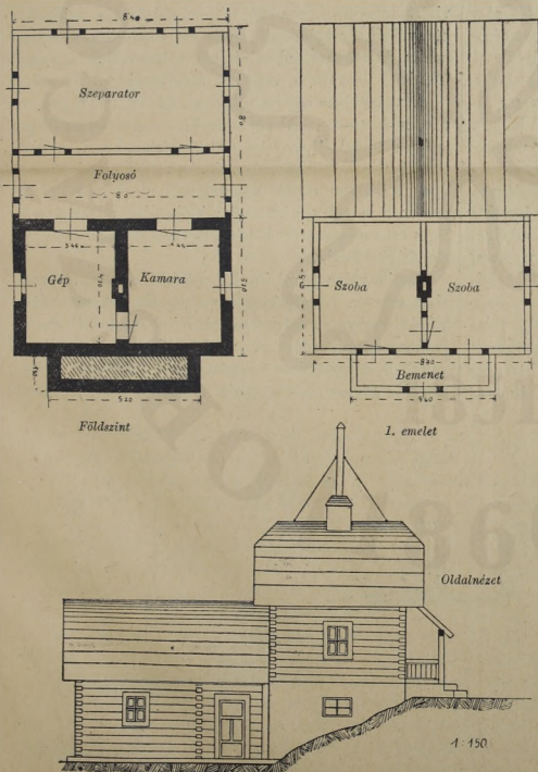
10. ábra. Mensesili tanya és gépház tervrajza.
