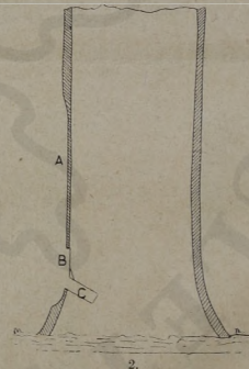
7—8. kép. Német gyantacsapolás fűrt gyűjtőgödörrel. A az elhalt kéregtől megtisztított rész, B hajk, C gyűjtőgödör. (Erdészeti Kísérletek 1917. évi 1—2. füzetéből.)
