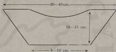
6. kép. Pléből készült kötény az amerikai gyantacsapoláshoz. (Az Erdészeti Kísérletek 1917. évi 1–2. füzetéből.)
