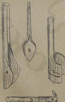
12. kép. Pinus-félék csapolásához szükséges szerszámok. A Kúpos véső a gyűjtőgödörhöz, B vaskanalát a balszam kiadásához, C íves véső a pléhlap berakásához, D kaparó a gyanta gyűjtéséhez. (Az Erdészeti Kísérletek 1917. évi 1—2. füzetéből.)
