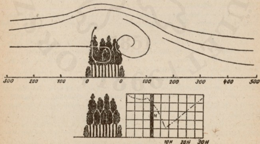
A szél sebességének csökkentése erdősávval
