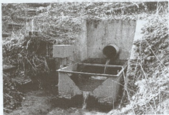
Elektronikus adatgyűjtővel felszerelt mérőbúka az egyik részvízgyűjtőben.
