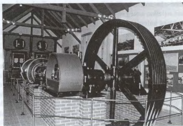
A lenti fűrészüzem gőzgépe egykor áramfejlesztő generátort is működtetett a fűrészgépek mellett. (A képek Szakács László felvételei.)
