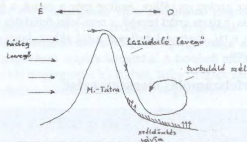
"A tátrai bóra" mozgásának vázlata nyugati irányból tekintve.
