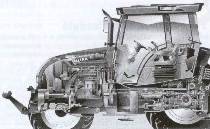
Az erdészeti célra is alkalmas, TwinTrac kormányzási rendszerű VALTRA N traktortípus szerkezeti ábrája. /Prospektus-kép/
