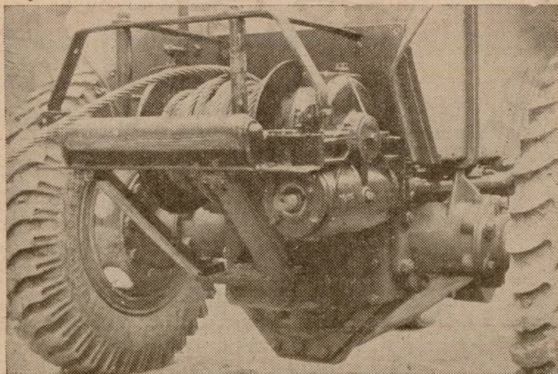
Traktorra szerelt csörlő: a gánti fakitermelés egyik fontos eszköze (Kaufmann József a Pest megyei erdőgazdaság géptelep igazgatójának útjása)
