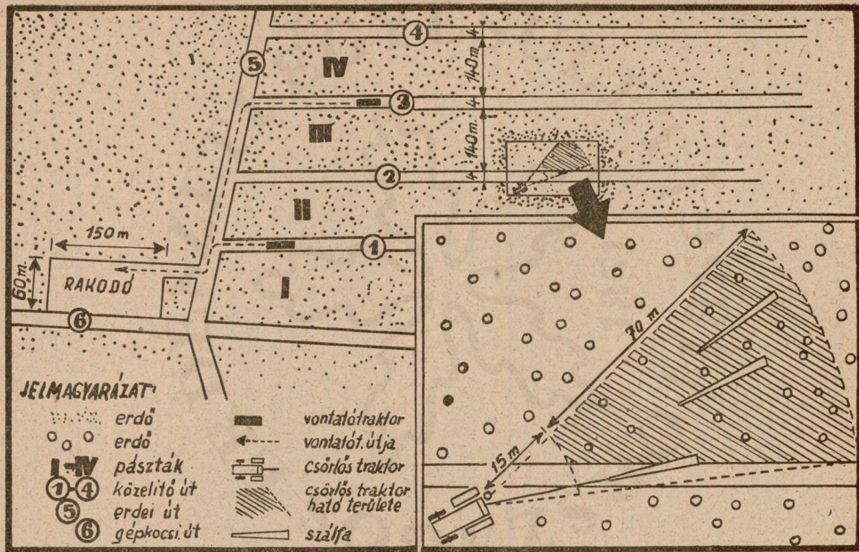
A gánti vágásterület helyszínrajza és a csőrös traktor munkaterülete
