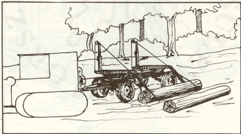
11. ábra. Oldalról történő felterhelés
