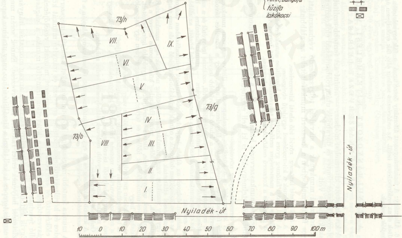
3. ábra. A pásztákra osztott vágésterület és a rakodó utak elhelyezkedése
