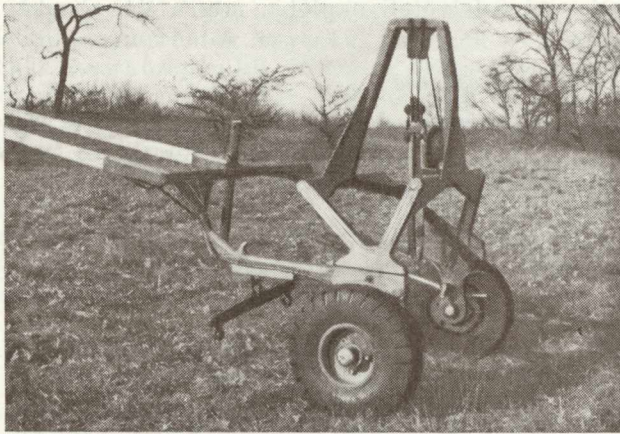
7. ábra. Közelítő kerékpár rönkadapterrel
