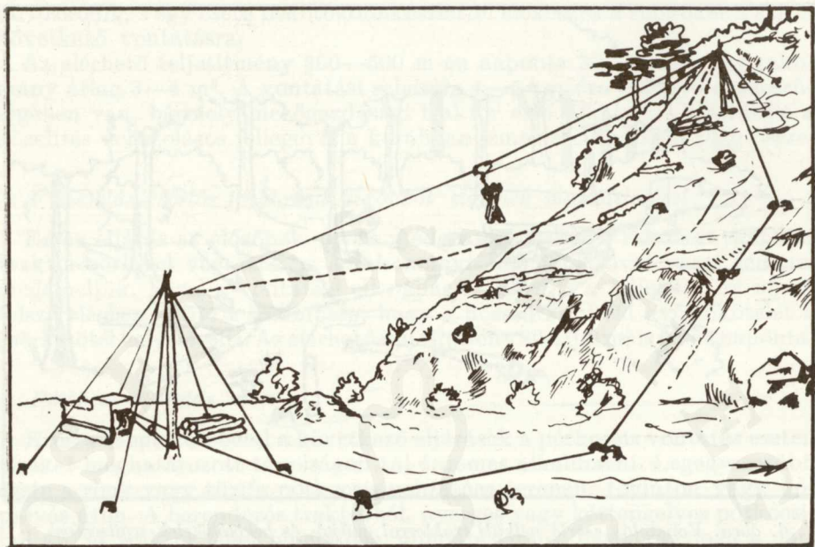
5. ábra. Közelítés a traktorcsörlőnek a tartókötelet mozgató kötélpálya kötélrendszerébe való kapcsolódásával
