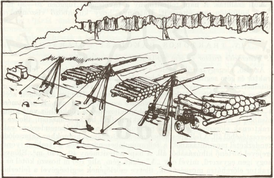
8. ábra. Felterhelés traktor és gém segítségével több máglyáról
