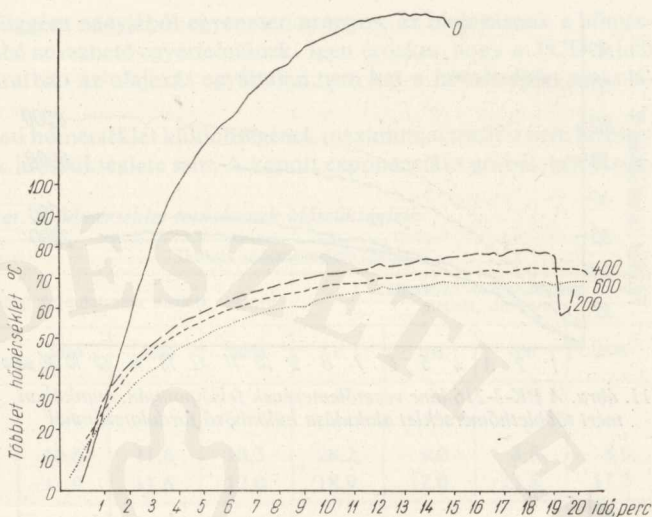
8. ábra. A PRH-11 lánc vezetőlemeze felső pontjában mért üresjáratú többlethőmérséklet alakulása különböző olajadagolásnál
