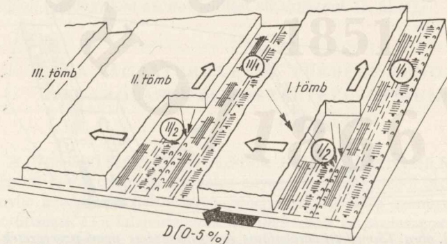
5. ábra. Tő melletti darabolásos és készletezéses munkaszervezet esetében a vágásterület térbeli rendje, ha minden művelet ugyanaz a munkaspár végez (szerk. Szász)
