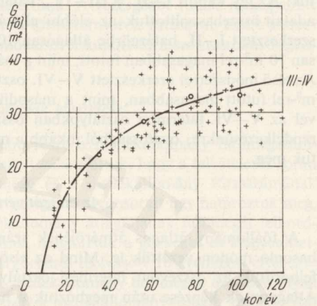
5. ábra. A III. és a IV. fatermési osztály főállománya körlapösszeg görbéjének szerkesztése az alapadatokkal
