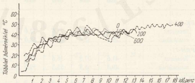
10. ábra. A PCU-1 lánc vezetőlemeze felső pontján, munkában mért többlethőmérséklet alakulása különböző olajadagolásnál
