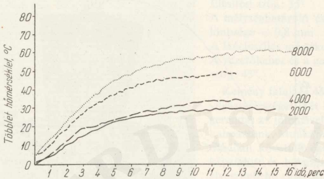
11. ábra. A BK-3-216 lánc vezetőlemezőnek felső pontján, munkában mért többlethőmérséklet alakulása különböző fordulatszámnál
