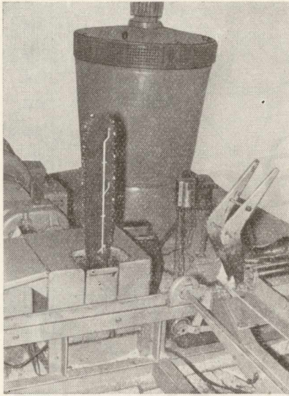
6. ábra. A termoelemek elhelyezése a kísérleti vezetőelemek egyikén
