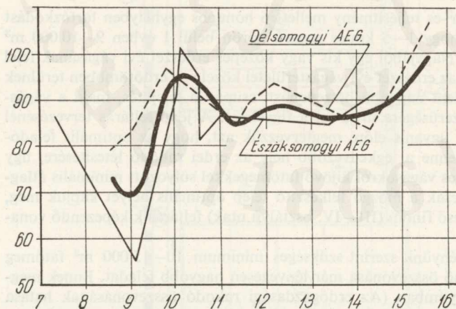
9. ábra. Az összes szállítási költség alakulása összevonás után a gépkocsi szállítási távolság függvényében
