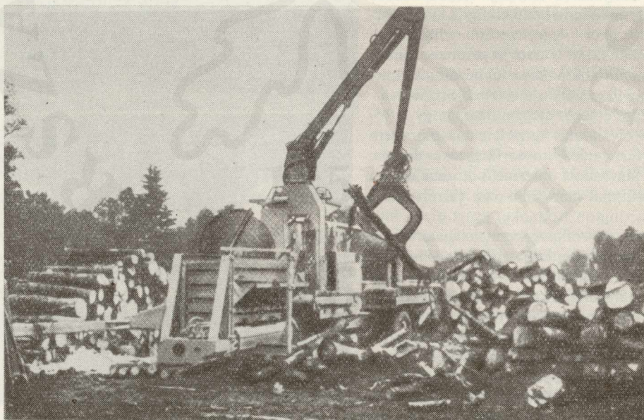
3. ábra. „Nesco” mozgó felkészítő gépsor. (Canadian Forest Industries 1967. July nyomán)
