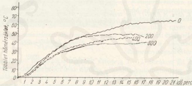
12. ábra. A BK-3-216 lánc vezetőlemezőnek felső pontján, munkában mért többlethőmérséklet alakulása különböző olajadagolásnál
