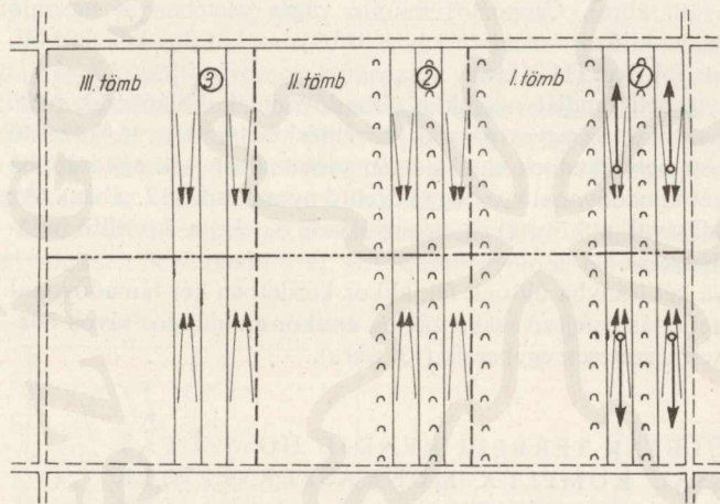
14. ábra. Hosszúfás közelítéssel komplex munkaszervezetek esetében soros telepítésű állományok gyérítésének térbeli rendje vízszintes és enyhe lejtésű terepen (szerk. Szász)
