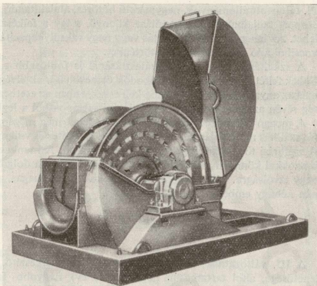
6. ábra. „Soderhamn Chipper” aprítékkészítő gép
