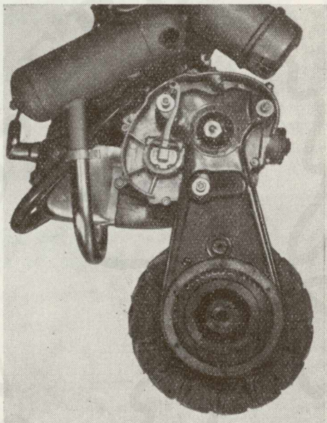
3. ábra. A motoroskapa kerék meghajtása
