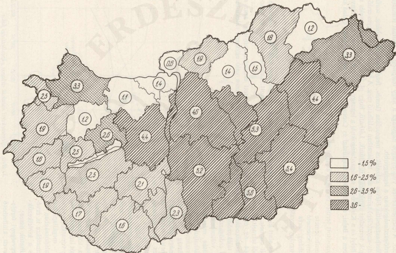
4. ábra. A csemetetermelési ágazat részesedése az összes ágazatok együttes termelési értékéből erdőgazdaságonként
