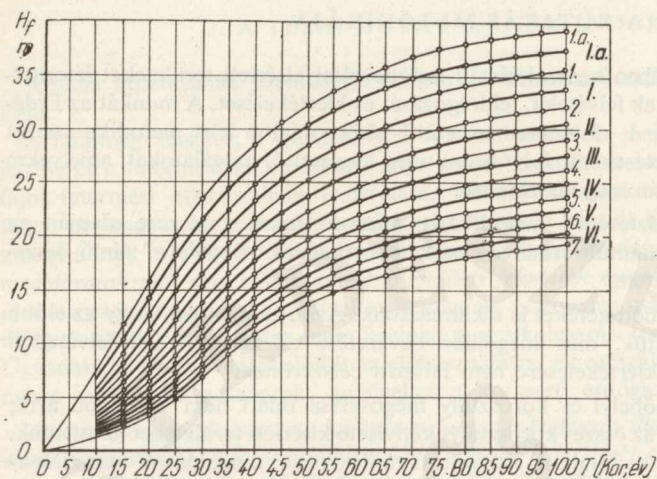
I. ábra. Az egyes fatermési osztályok felsőmagassági közép- és határ- görbéi
