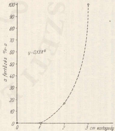
2. ábra. A fertőzések vastagsági kategóriák szerinti elrendeződésének modellje
