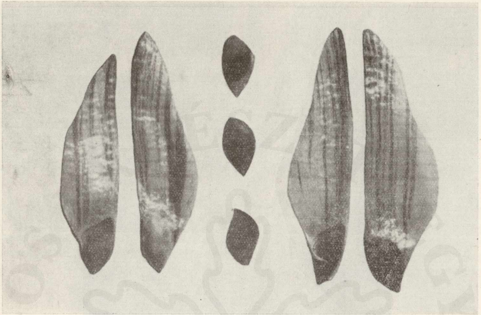
3. ábra. Az 1—4 jelű klón csikos szárnyú magja
