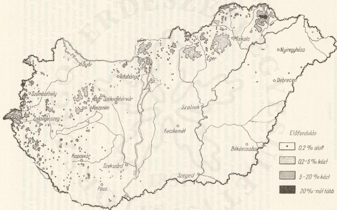
1. ábra. A lucfenyő elterjedése
