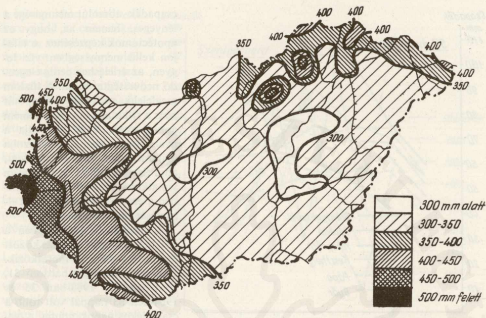
2. ábra. A csapadék nyári félévi összegének területi eloszlása mm-ben. 50 évi átlag (1901—1950) (Hajósy nyomán)
