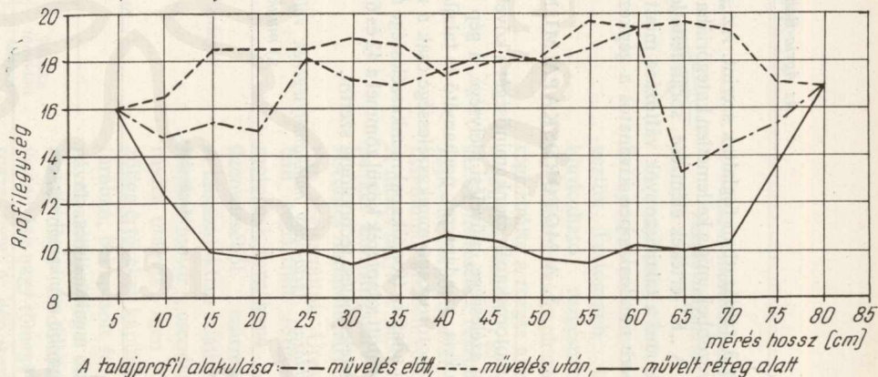
6—7. ábra. A talajprofil alakulása
