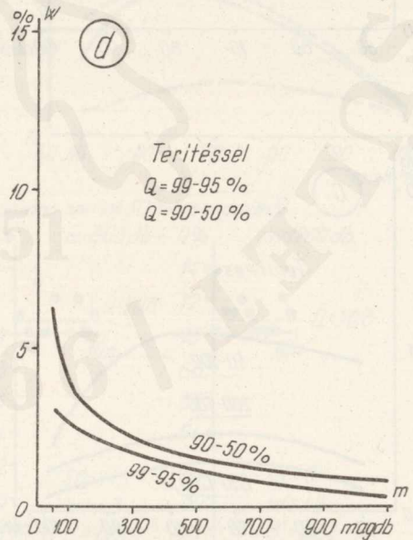
3. ábra. Feketefenyő: variációs szélesség a minta magdarabszám függvényében
