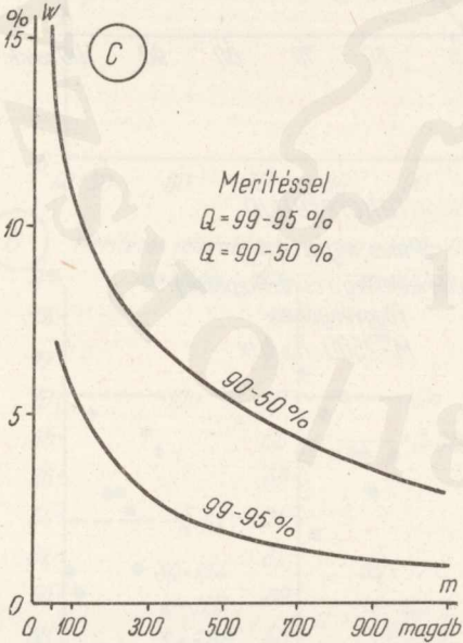
3. ábra. Feketefenyő: variációs szélesség a minta magdarabszám függvényében
