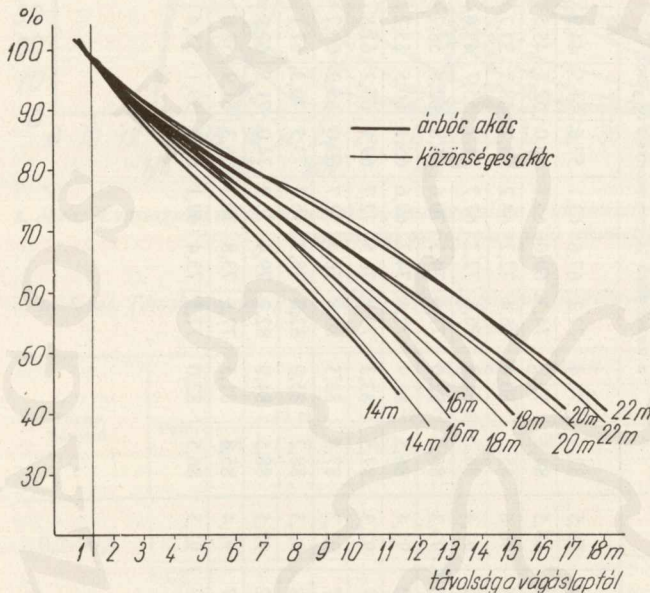
2. ábra. Az árbc és közönséges akác törzsalakSORAI a fmagasság függvényében
