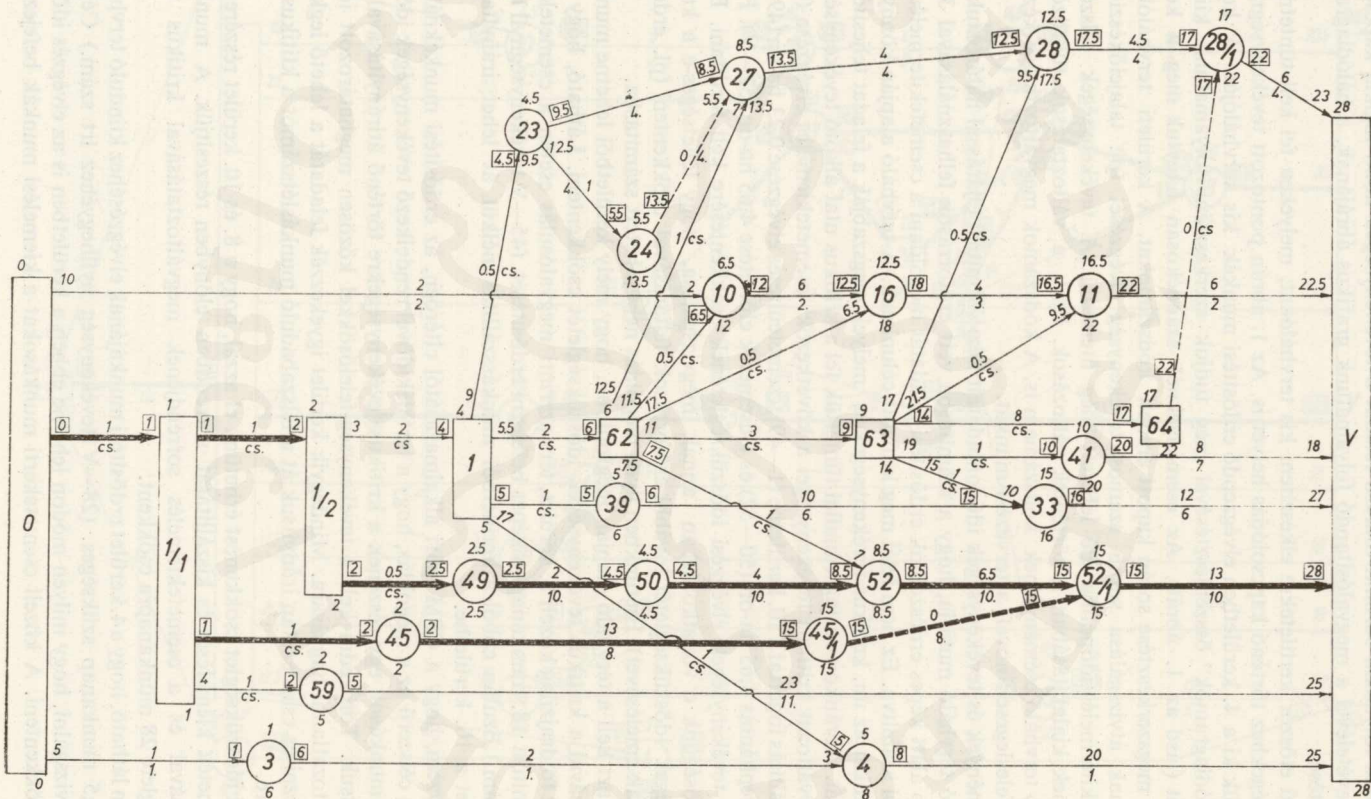
2. ábra. A 2. tervváltozat hálódigramma
