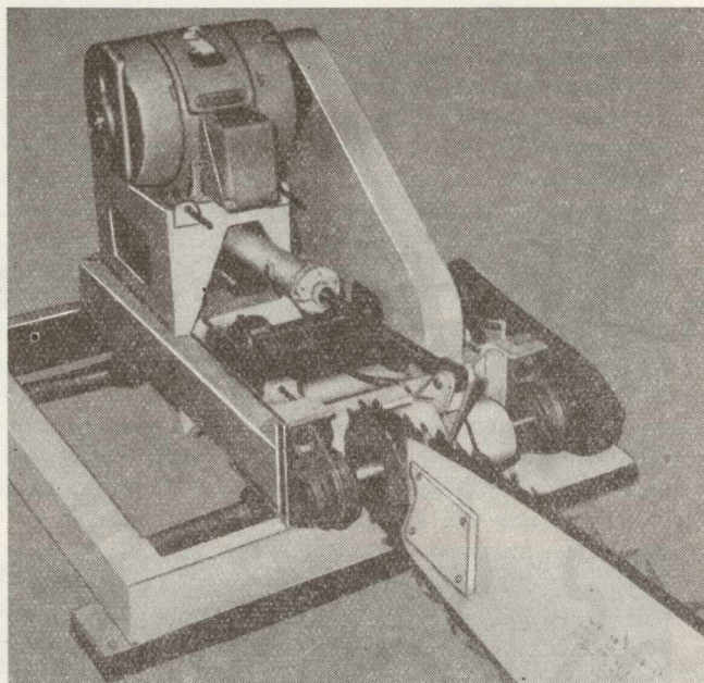
5. ábra. „Brute” daraboló láncfűrész
