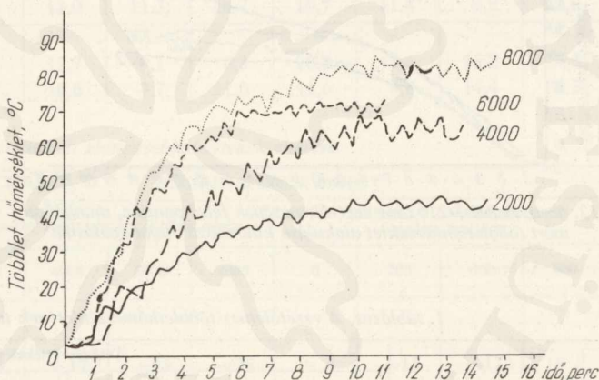
9. ábra. A PCU-1 lánc vezetőlemeze felső pontján, munkában mért többlethőmérséklet alakulása különböző fordulatszámmal
