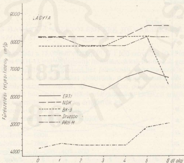
2. ábra. Az egyes láncok fűrészelési teljesítményének alakulása nyárnyáiban, különböző olajadagolás mellett
