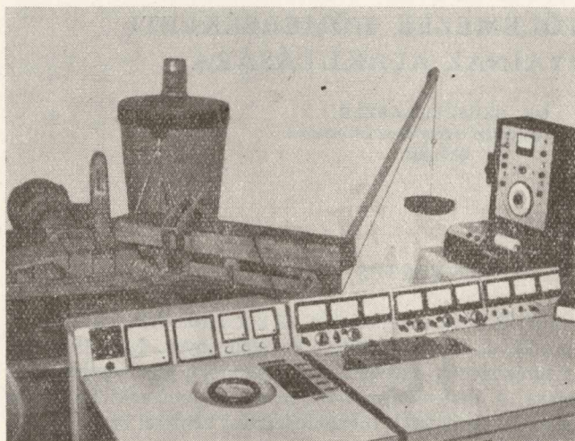
1. ábra. A fűrészláncvizsgáló próbapad
