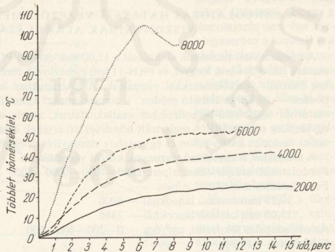
7. ábra. A PCU-1 lánc vezetőlemeze felső pontján mért üresjáratú többlethőmérséklet alakulása
