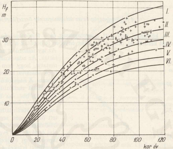
1. ábra. A kísérleti területek felsőmagassági adatainak elhelyezkedése a szórásmezőben
