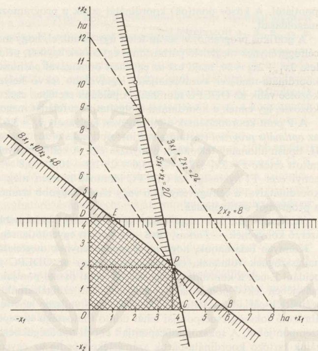
1. ábra. Optimális erdősítési program készítése grafikus módszerrel
