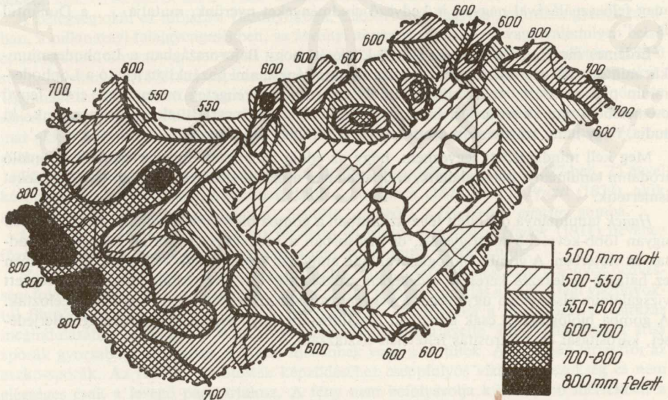
1. ábra. A csapadék évi összegének területi eloszlása mm-ben. 50 évi átlag (1901—1950) (Hajósy nyomán)
