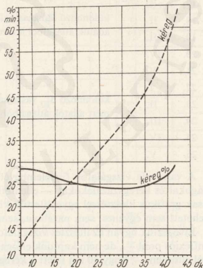
4. ábra. Az akác kéregvastagsága és kéreg %-a grafikus kiegyenlítés alapján
