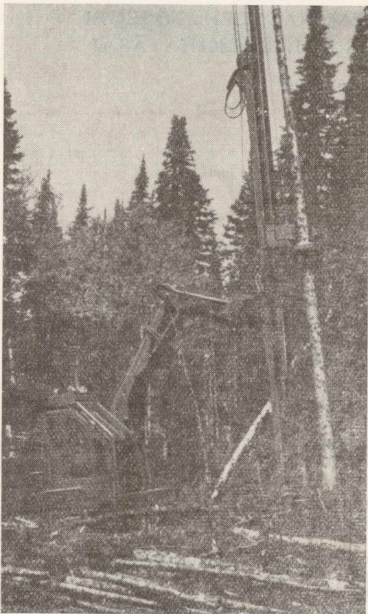
1. ábra. Beloit harvester fakitermelőgép. (Canadian Forest Industries 1967. July nyomán)
