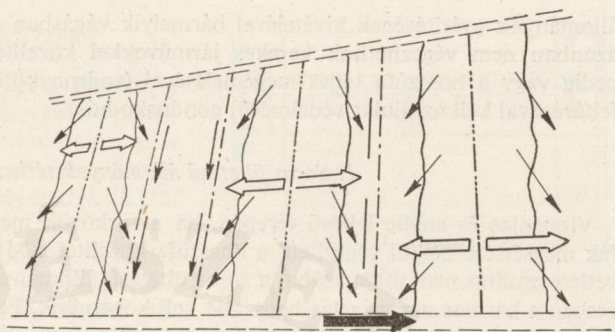
13. ábra. Vonalas felújítóvágás térbeli rendje, ha a támadóvonalról a vágással két irányba haladunk (szerk. Szász)
