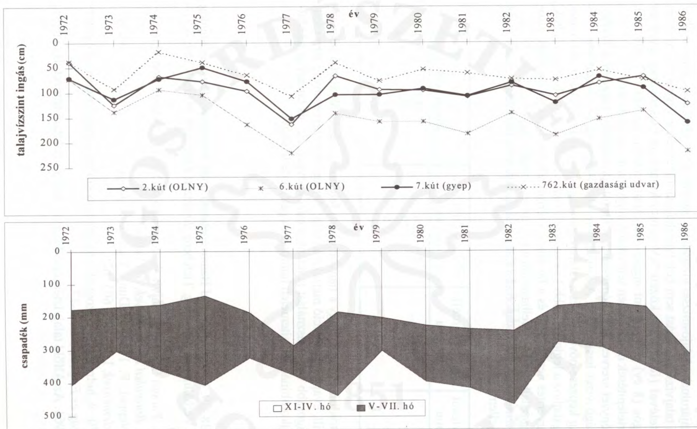
4. ábra. Lajosmizsei olasznyárasban az éves talajvízszint ingás változása
