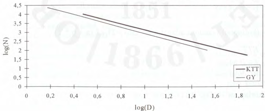
3. ábra. Log(D) és log(N) összefüggése a két fajra
