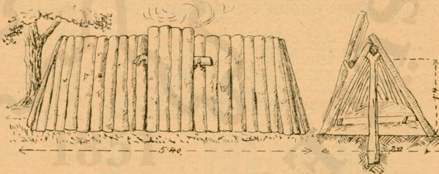
(2. ábra.) Vadászkunyhó hasítványokból hat személyre.
