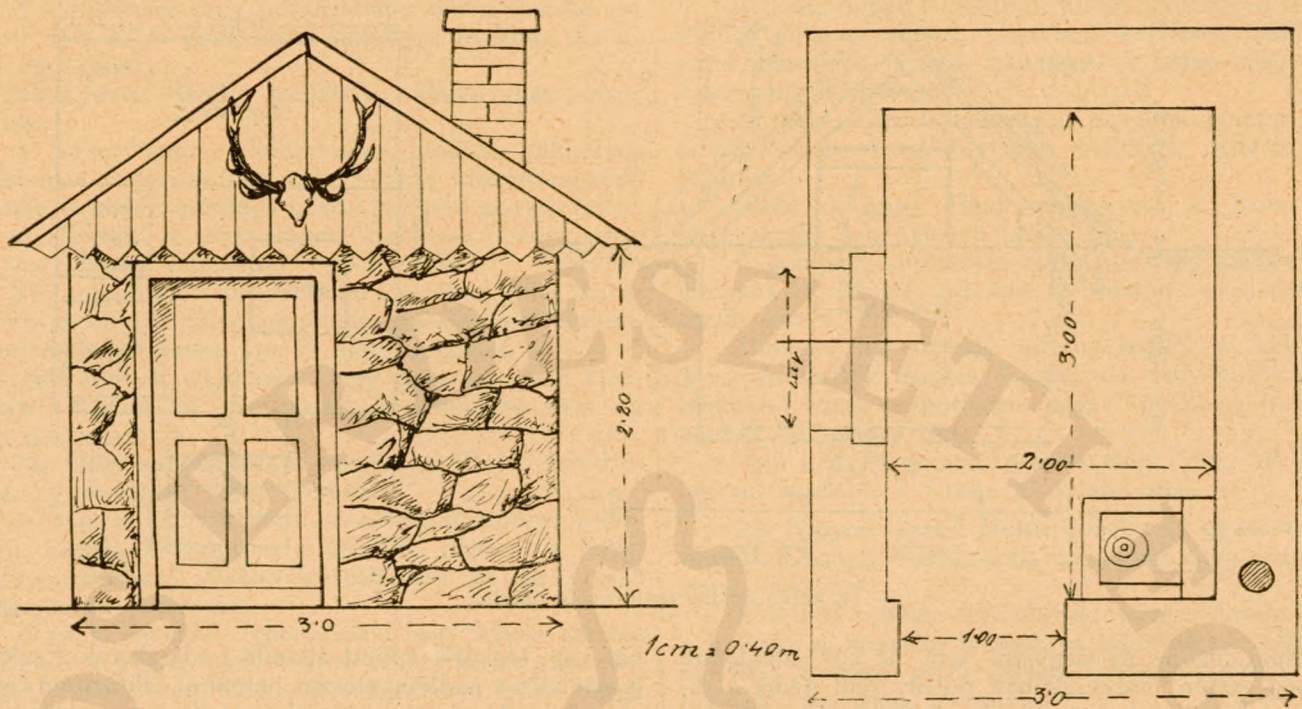
(3. ábra.) Egyszobás, terméskövekből épített vadászlak.
