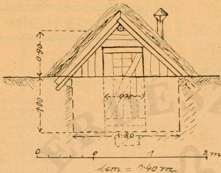
(1. ábra.) Földbe ásott vadászkunyhó.
