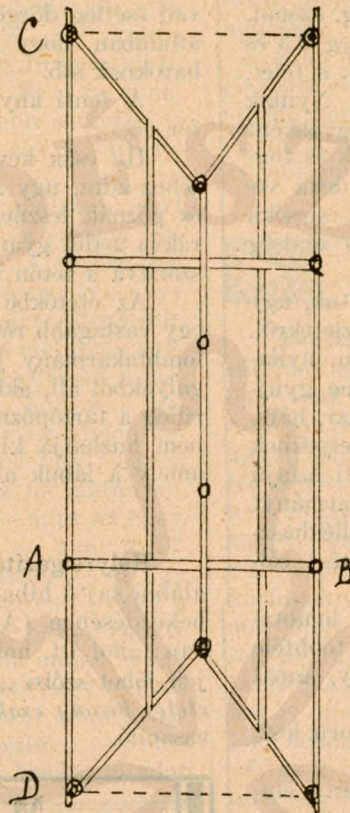
2. Alaprajz felülről nézve a hevederekkel és gerinc léccel.
