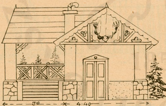
(4. ábra.) Szoba, konyha és verandás vadászlak.
