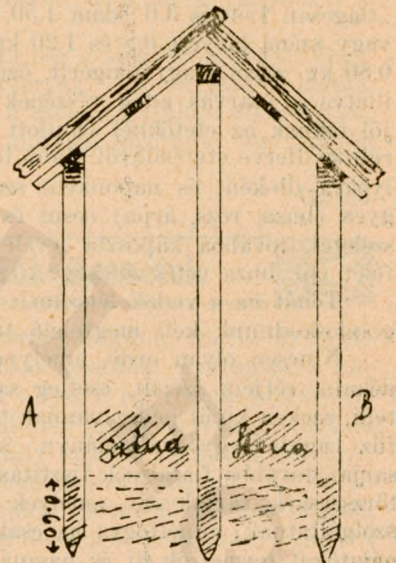
3. Az etető kereszt metszete. (A - B)
