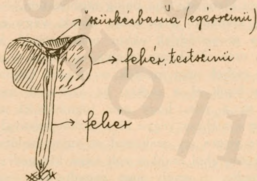
(Nyulfülegomba tollrajza.)
