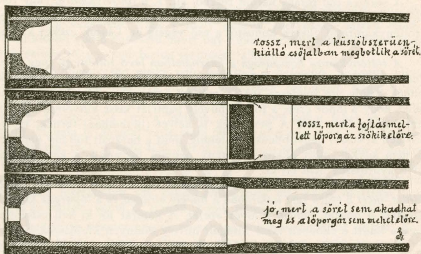
Konusfűrási módok.
