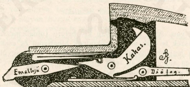
Anson & Deeley lakat.
