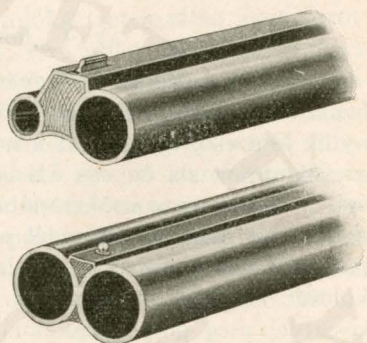
Csővégekiképzés (csősin)
