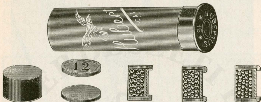
Magyar „Hubertus“ hüvely, fojtások és becsavarási módok.
