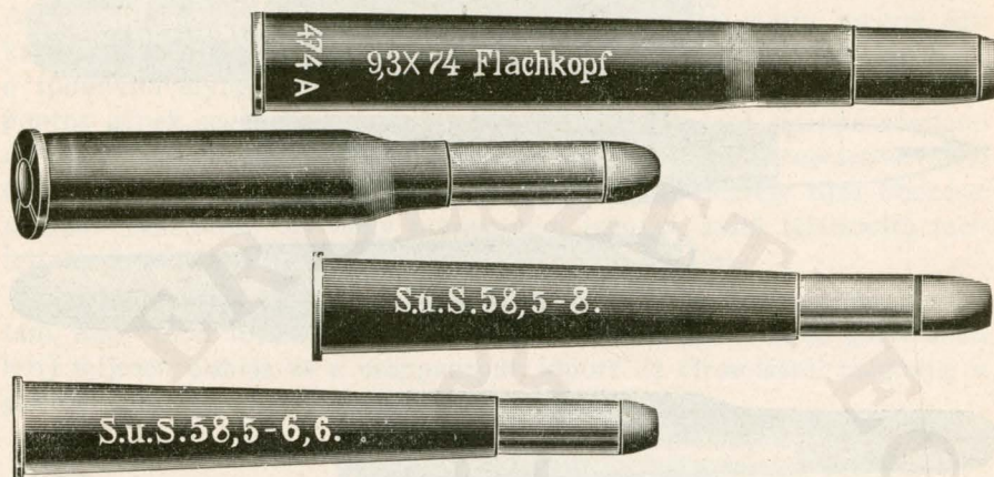
Nagyvadra való töltények fémburkolattal. B) peremmel ellátva.
