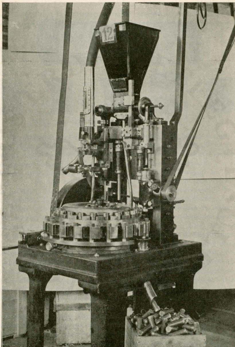
Töltőgép a magyaróvári vadásztölténygyárban.
