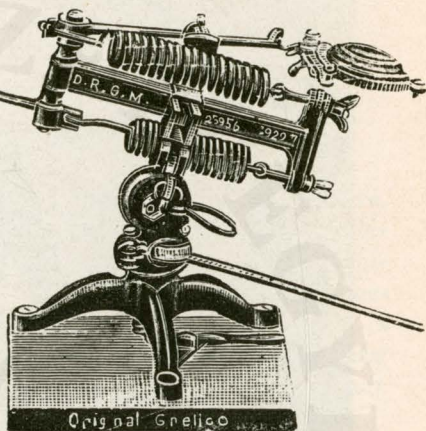
Aszfaltgalambdobógép
