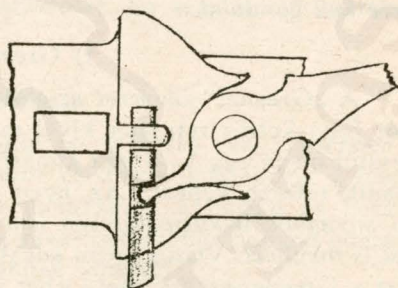
Greener-závarzat.
