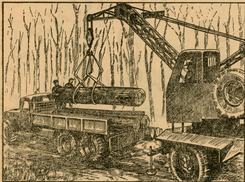
A rakodók géppel emelik autóra a rönköket
