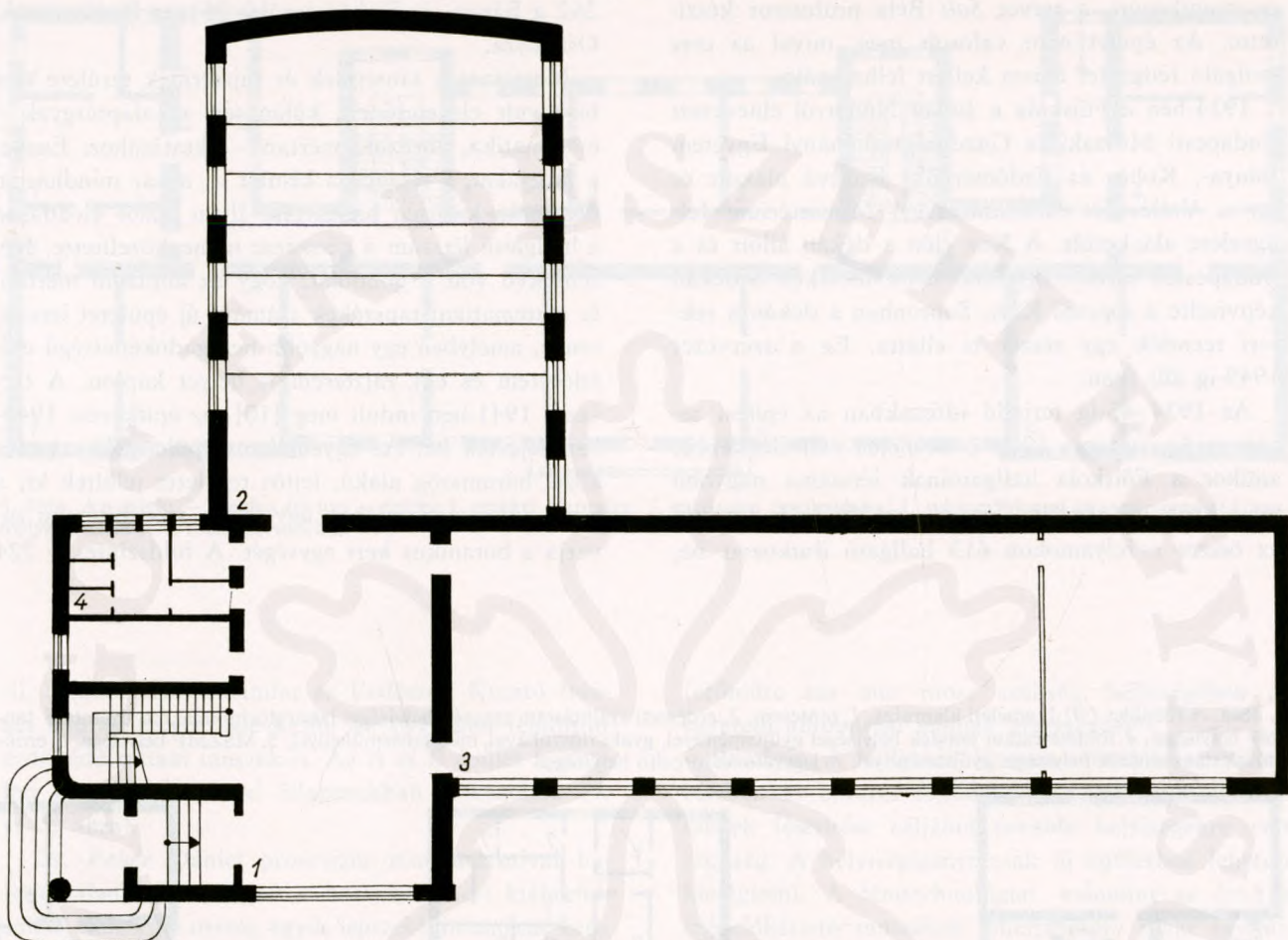
6. ábra. Az ábrázoló mértani és matematikai tanszékek helyiségeit befogadó épület földszinti alaprajza. 1. előcsarnok, 2. tanterem, 3. rajzterem, 4. előadói szoba
