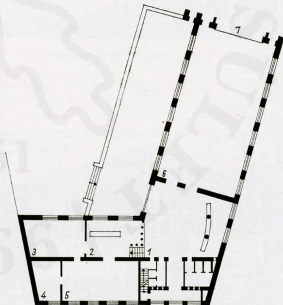
10. ábra. A KISZ-ház földszinti alaprajza 1. előcsarnok ruhatárral, 2. büfé, 3. TV-szoba, 4. olvasó, 5. klubszoba, 6. előadóterem, 7. színpad és tartozéka
