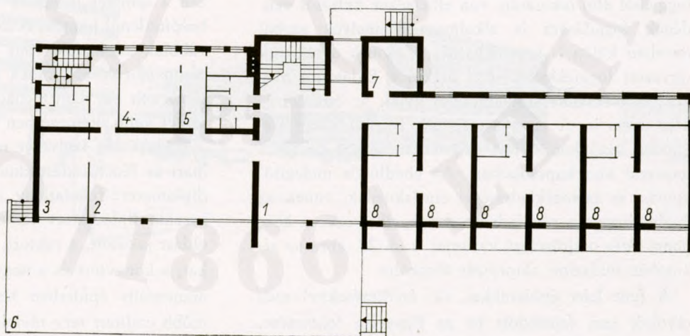
23. ábra. Az Egyetem keszthelyi alkotóháza földszinti alaprajza. 1. előcsarnok, 2. étkező-nappali, 3. TV-szoba, 4. melegítőkonyha, 5. mosogató, 6. terasz, 7. iroda, 8. lakószobák
