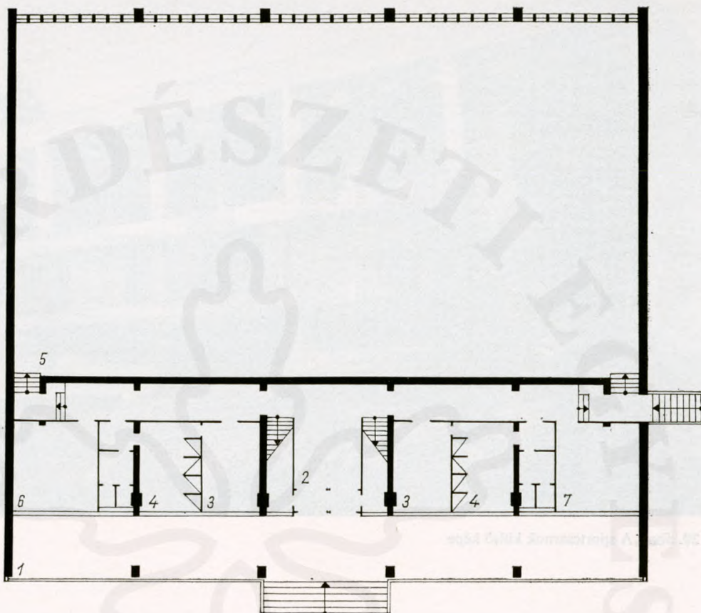
19. ábra. A sportcsarnok földszinti alaprajza 1. nyitott bejárati csarnok, 2. előtér, 3. öltöző, 4. fürdő, 5. csarnok, 6. hőközpont, 7. szertár
